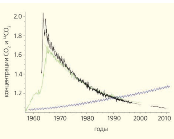
Рис.1. Изменение атмосферных концентраций радиоуглерода и \text{CO}_2 по отношению к их уровням 1950 г. Данные измерений радиоуглерода (чёрная кривая для Северного полушария, зелёная — для Южного) взяты из работ [8, 9, 10]. Хорошо известные данные измерений атмосферной концентрации \text{CO}_2 (синяя кривая) также нормированы на уровень 1950 г. Колебания всех экспериментальных зависимостей происходят с периодом 1 год, это сезонные вариации. Штриховая чёрная линия на кривой ^{14}\text{C} — экспонента с характерным временем 13.5 лет, штриховая зелёная линия — экспонента с характерным временем 16.7 лет. Штриховая синяя линия \text{CO}_2 — сглаженные ежегодные средние.
