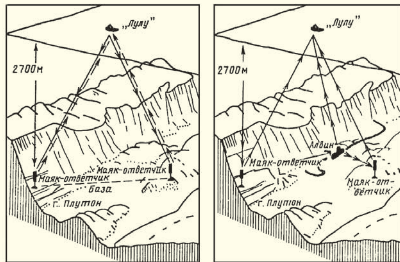
Рис.5. Схема координации подводных исследований на полигоне «ФАМОУС» [3].
