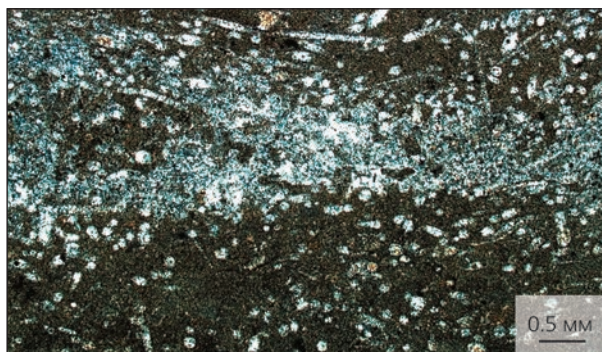
Рис.5. Микрофотография микрозернистых битуминозных известняков с обильными остатками радиолярий и редкими спонгулами губок из верхней части циклитов.
