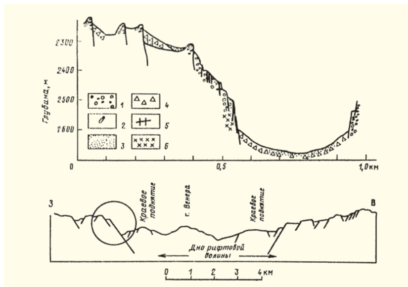
Рис. 7. Геологический разрез на склоне рифтовой долины по наблюдениям с глубоководного обитаемого аппарата «Алвин» [3]. Вверху — геологический разрез внутренней стены западного склона, внизу — поперечный профиль рифтовой долины и местоположение геологического разреза. 1 — подушки; 2 — валики; 3 — донные осадки; 4 — осыпи; 5 — дайки и силлы; 6 — брекчия.
