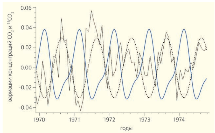
Рис.3. Сравнение сезонных колебаний концентраций радиоуглерода (черная ломаная и ее периодическая штриховая аппроксимация) и диоксида углерода на широте 48^\circ Северного полушария (синяя кривая). Они происходят практически в противофазе — по причине того, что максимум сжигания ископаемых топлив приходится на зимние месяцы Северного полушария, а затем газ \text{CO}_2 (максимум его концентрации достигается в феврале) заметно разбавляет атмосферный радиоуглерод.
