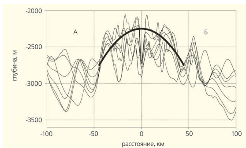
Рис.8. Осевой вулканический массив, расчлененный веером рифтовых долин.
