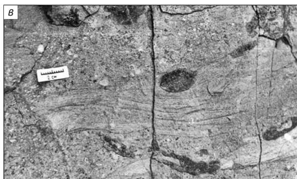
Рис.7. Характер отложений линзовидного тела: а — несортированные грубообломочные известняки с крупными экстракластами, б — крупный экстраклат светлого известняка с начальным размером не менее 0.5 м, в — крупный неокатанный экстраклат тонкослоистого известняка с кремневыми (черными) линзами. Длина ручки молотка 0.4 м.
